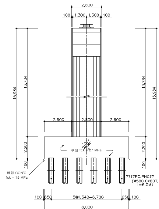
단 면 도 S=1:100
