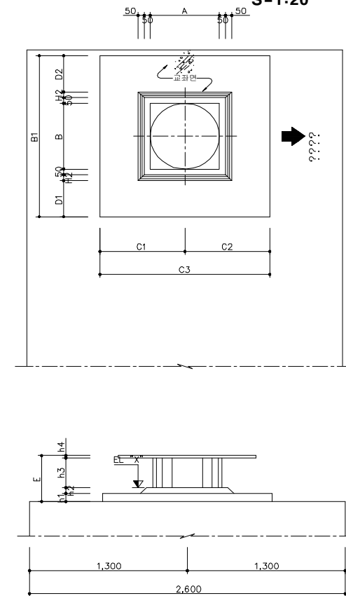
교량 받침 상세 S=1:20
