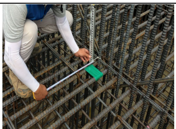
A2 기초 철근 조립 상태
