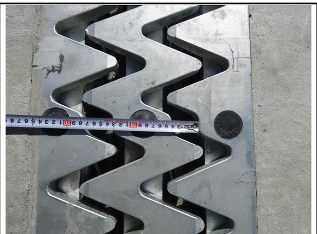
신축이음 P4 유간 측정
