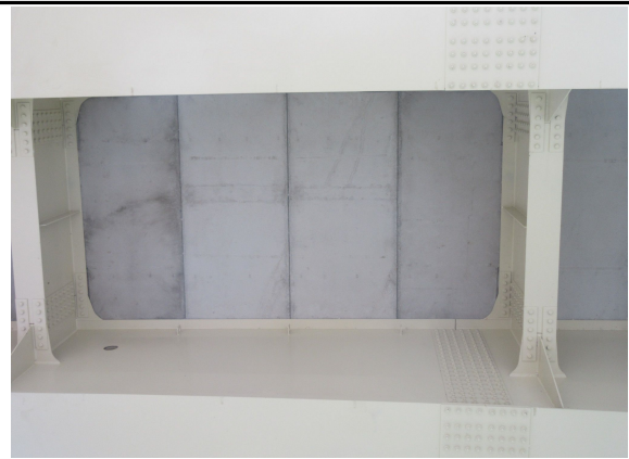
바닥판 하면(LB-DECK) 시공 상태 점검
