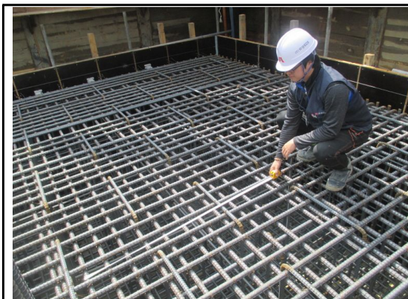
P6 기초 철근 배근 상태 측정
